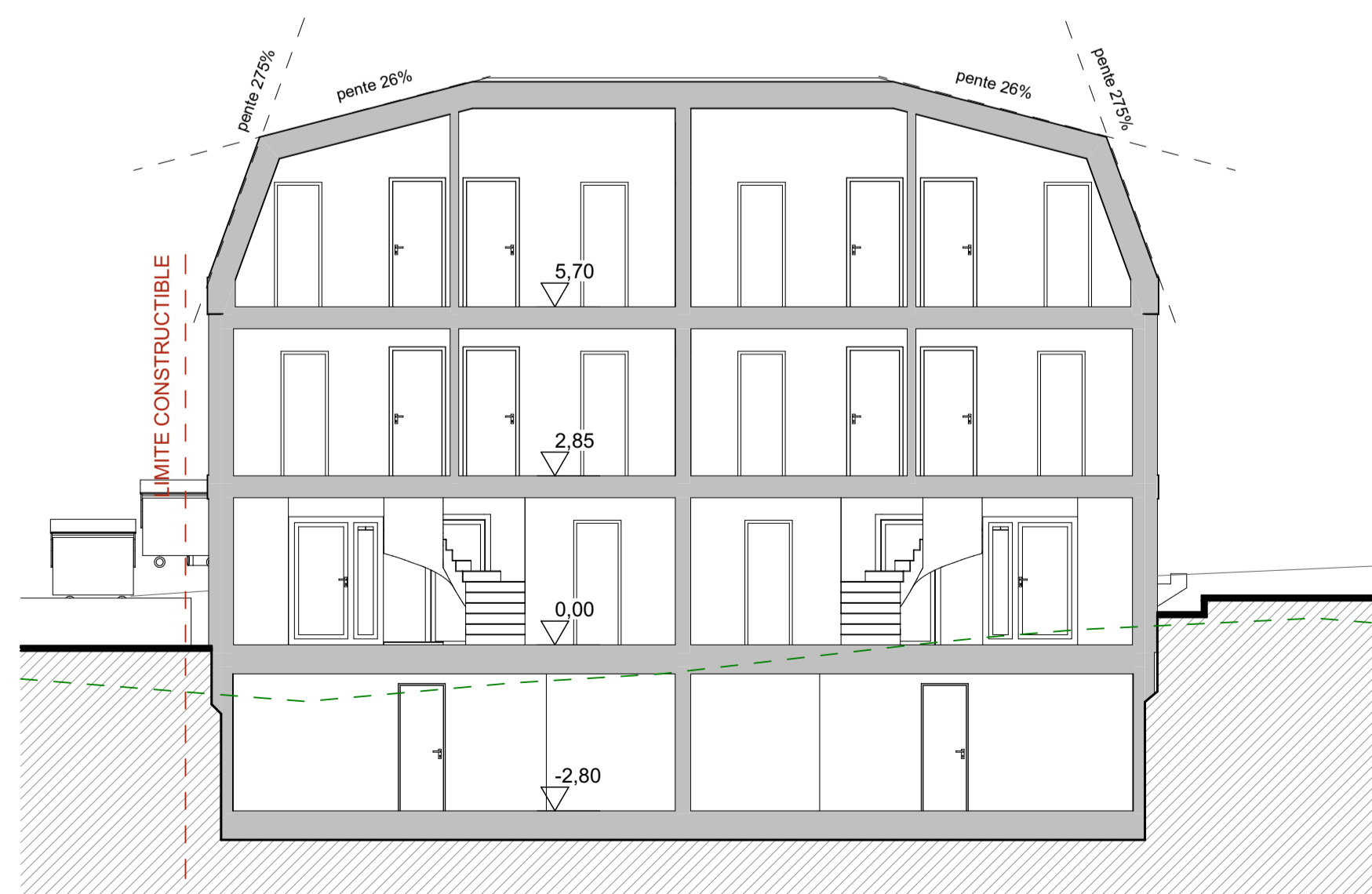
Coupe B 1:100
