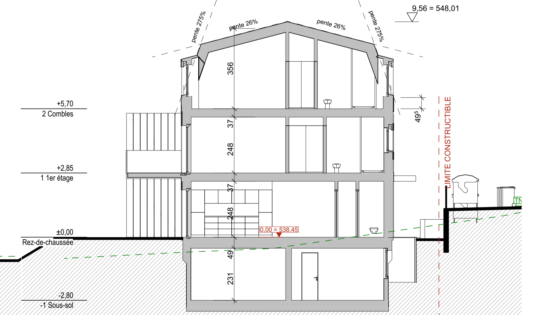
Coupe A 1:100
